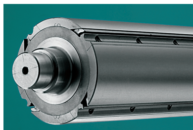
Option Planer shaft "MONOBLOC" with Torsa Knives Messerhobelwelle mit Torsa-Messern Вал "МОНОБЛОК" ножи Терса
